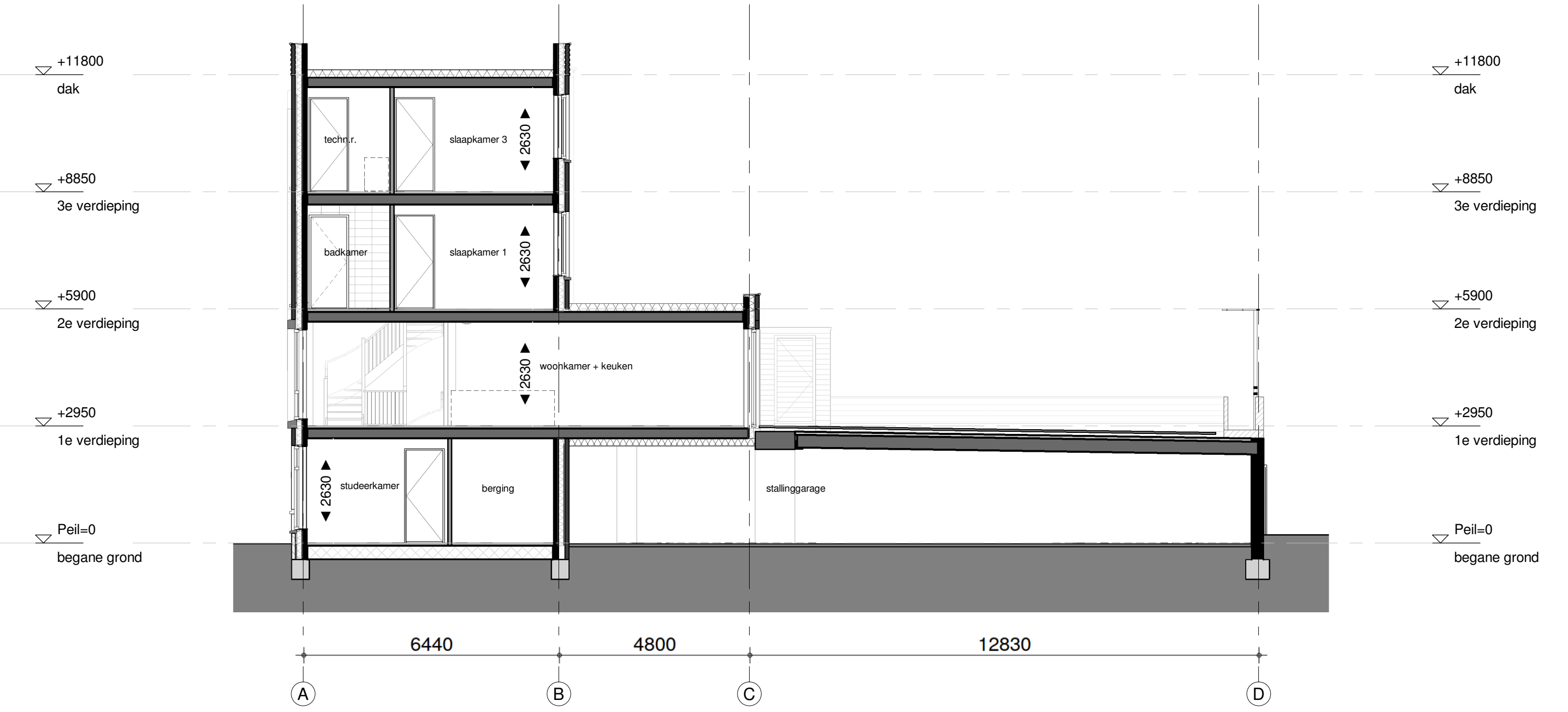
doorsnede 1 : 100
