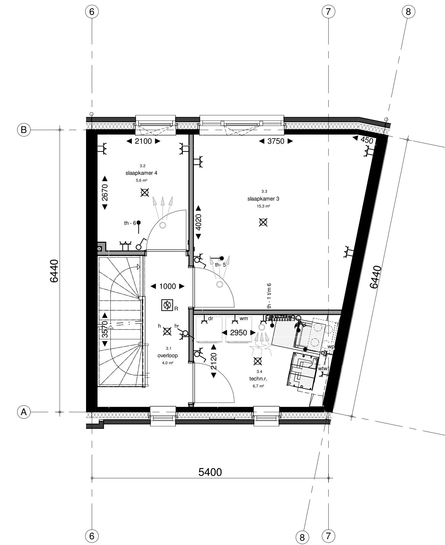
3e verdieping 1 : 50
