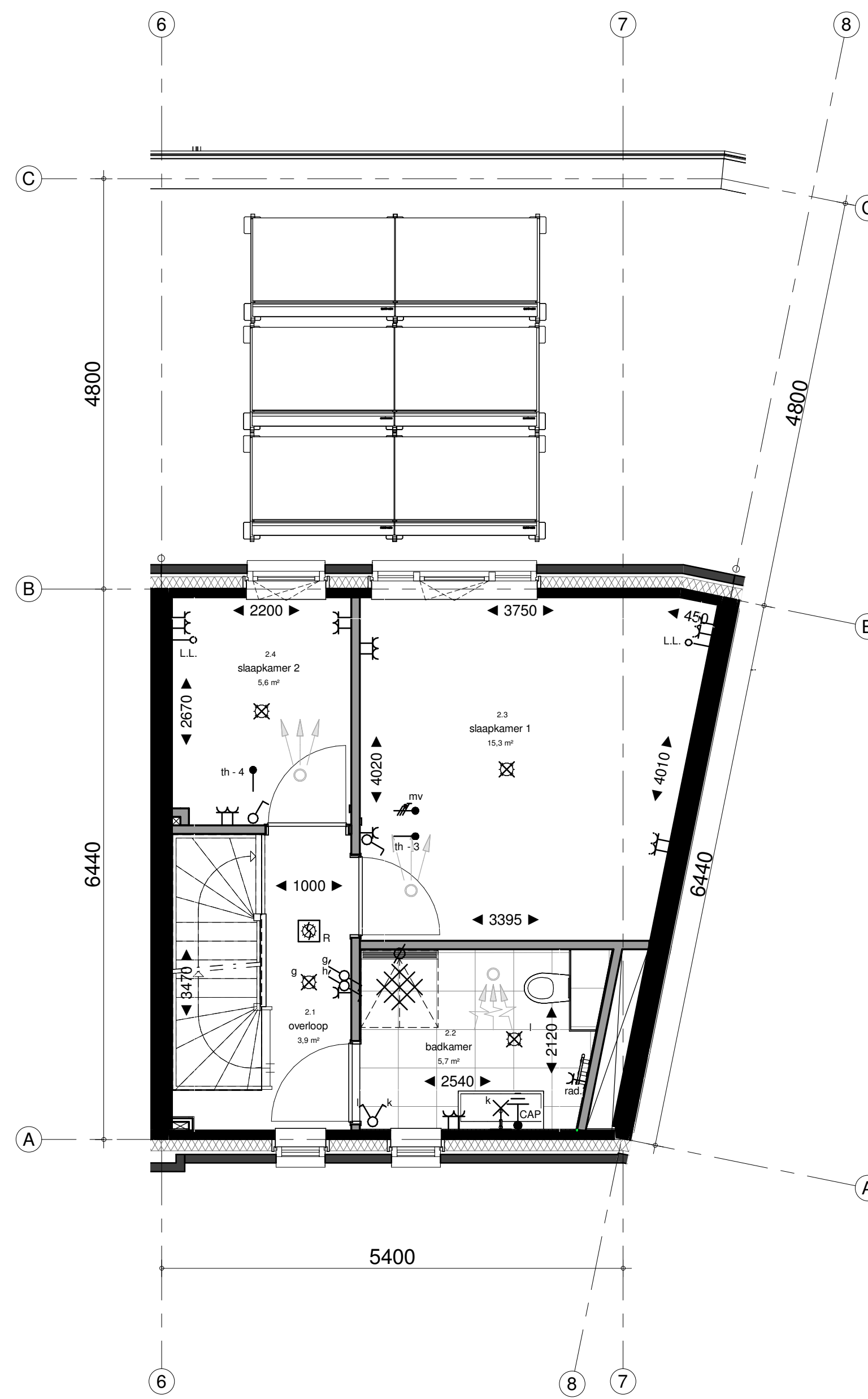
2e verdieping 1 : 50
